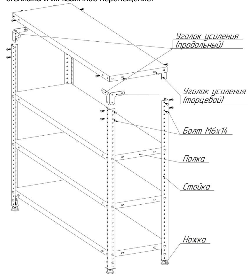
Рис. 2. Схема сборки складского стеллажа
